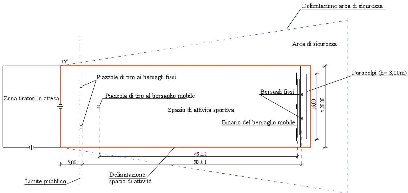
Fig. 1 Schema tipo - Area di attività sportiva
